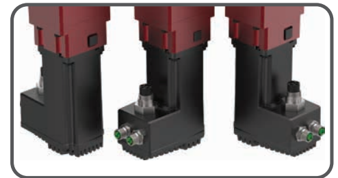
Motoranschlusspositionen können in 90°-Schritten gedreht werden
